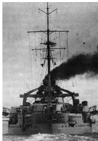
Heckansicht der „Rheinland“. Gut zu erkennen ist der hintere 280-mm-Geschützturm. Links ist einer der Seitentürme zu erkennen, ebenfalls mit zwei 280-mm-Geschützen, eine konstruktive Besonderheit, die es nur auf den Linienschiffen des „Nassau“-Typs gab und die sich nicht bewährte.
