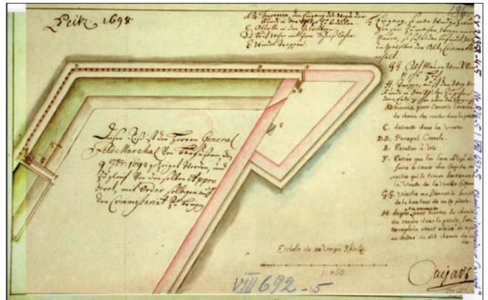
Einer der wenigen erhaltenen Festungsbaupläne von Cayart zeigt einen Änderungsbau in der Festung Peitz und ist mit 1698 datiert. Der Vermerk lautet, dass dieser Plan am 9. September 1698 dem Generalfeldmarschall Barfus gezeigt wurde.
