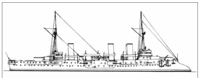
Seitenriss des französischen Kreuzers 1. Klasse „d’Entrecasteaux“, etwa 1896. 1927 wurde das Schiff (ohne Bewaffnung und Maschinen) an Polen verkauft. Foto: Archiv
