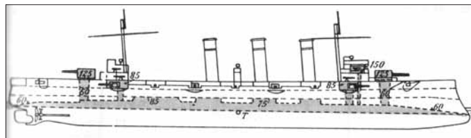
Seitenriss des Kreuzers mit der Anordnung der Artillerie und der Panzerung.
