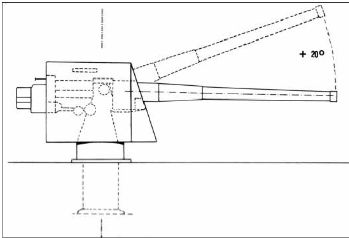
Während des 1. Weltkrieges würde die in Türmen untergebrachte Hauptartillerie (152 mm) des Kreuzers durch neue 130 mm-Geschütze mit Splitterschutz ersetzt.
